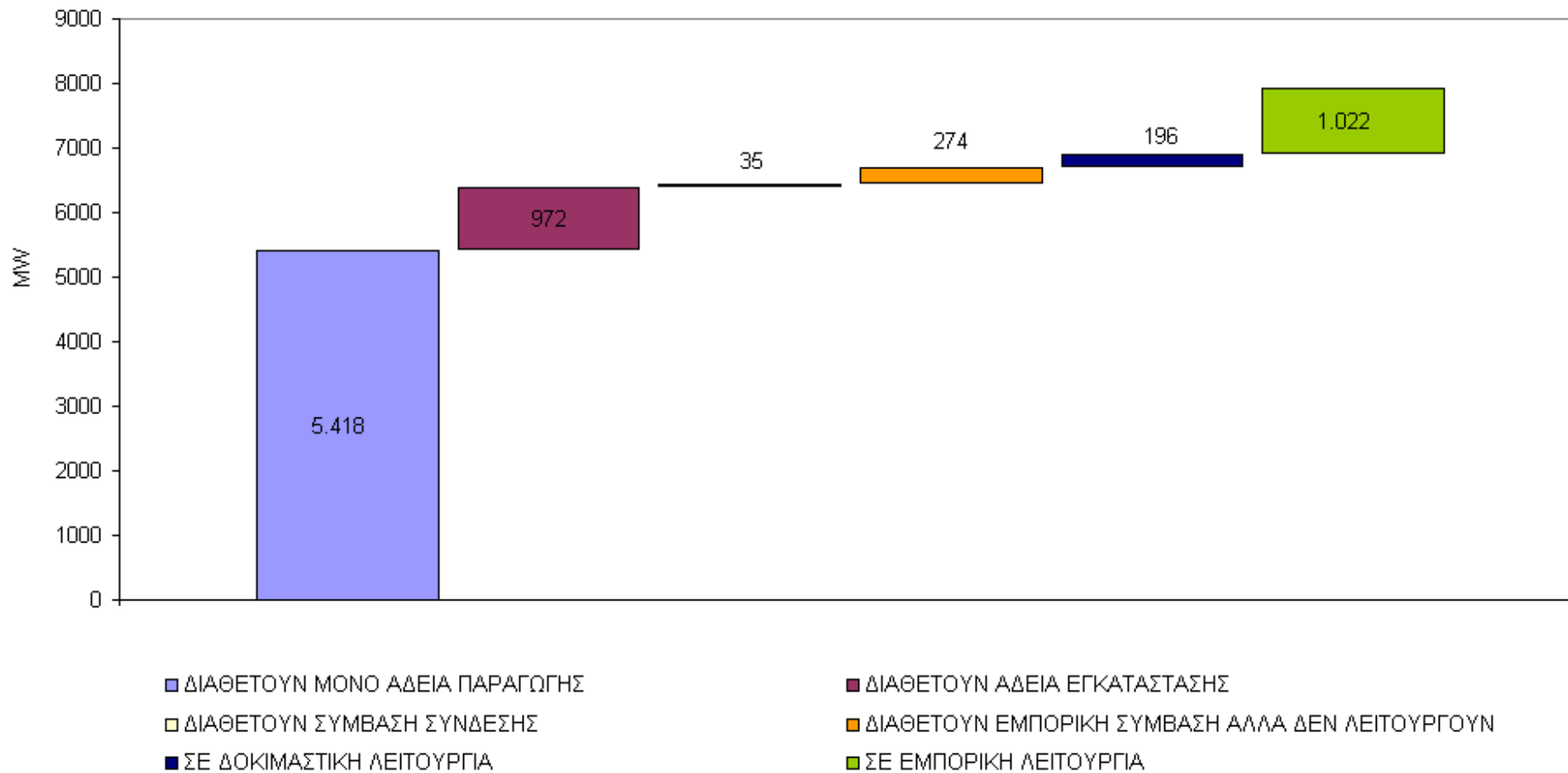
ΕΝΔΕΙΚΤΙΚΟΣ ΠΙΝΑΚΑΣ ΥΛΟΠΟΙΗΣΗ ΕΠΕΔΥΣΕΩΝ ΑΠΕ & ΣΗΘΥΑ ΣΤΟ ΔΙΑΣΥΝΔΕΔΕΜΕΝΟ ΣΥΣΤΗΜΑ (MW) 2009 (Άρθρο 9 Ν. 3468/06)
